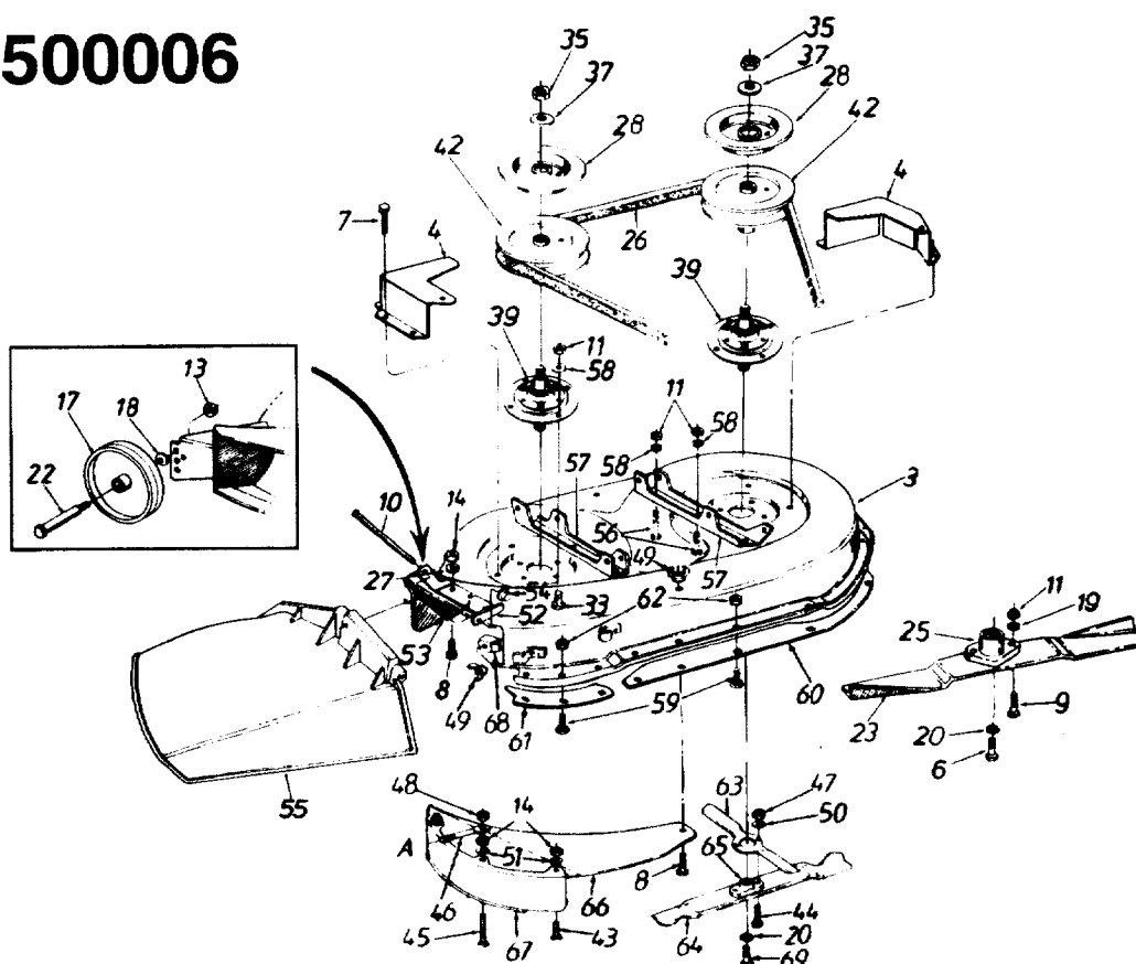
18 H.P. 42\"/>
